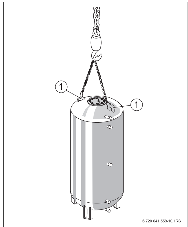
Рис. 5 Подъём краном
