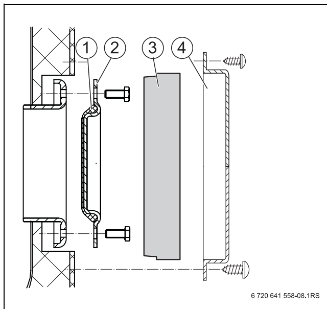
Рис. 14 Демонтаж крышки люка
