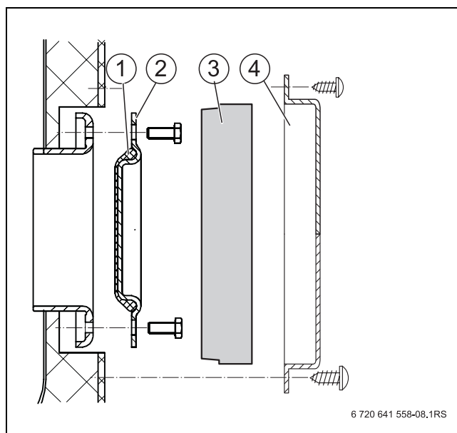
Рис. 17 Установка крышки люка
