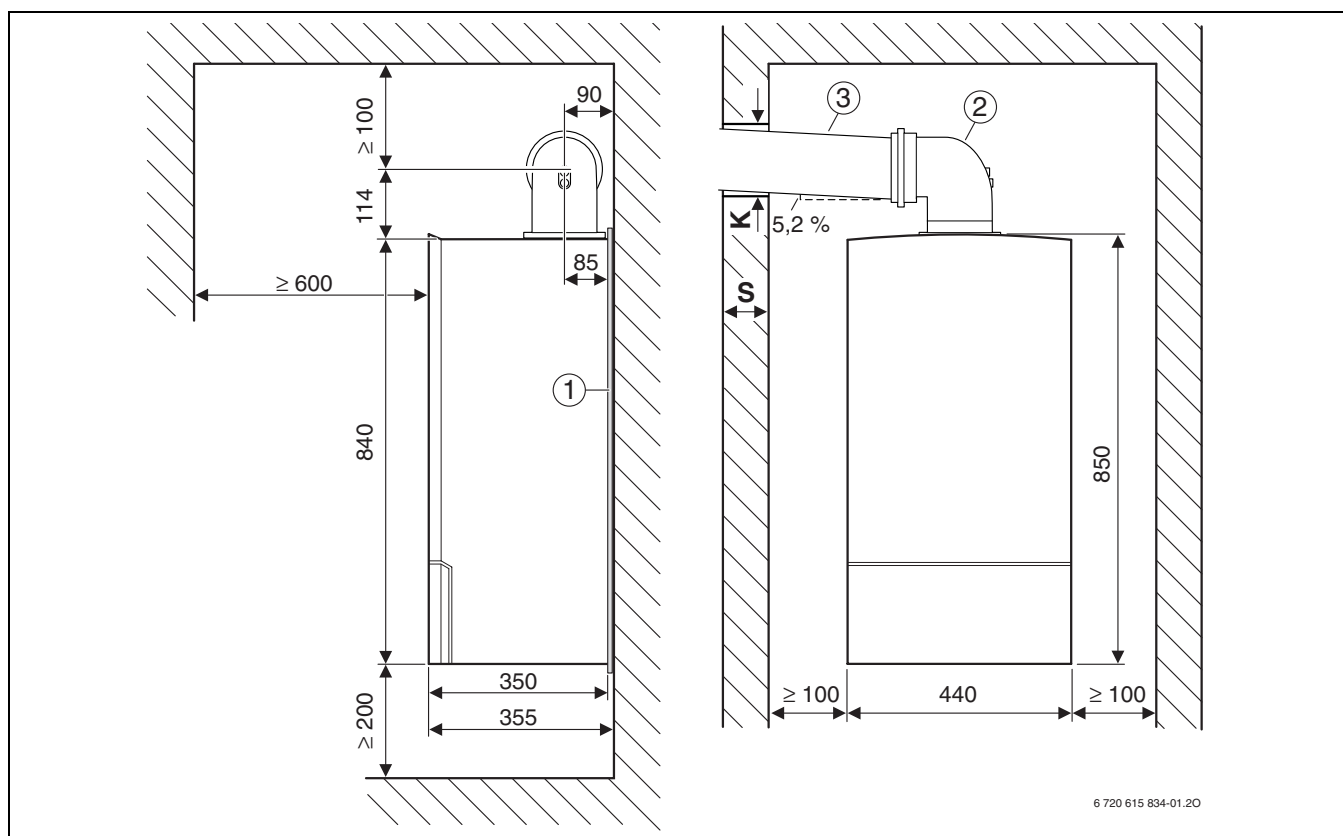
Рис 5 Отвод дымовых газов Ø 80/125 мм или Ø 80 мм
